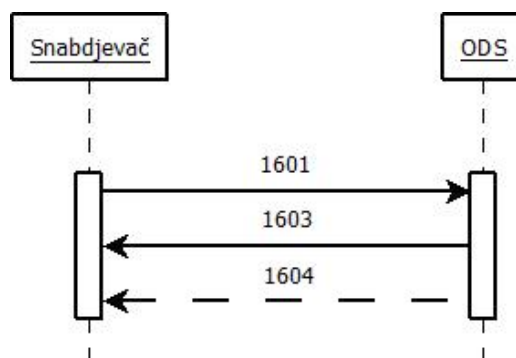
Slika 53: Sekvencijalni dijagram za varijantu procesa Isključenja mjernog mjesta na zahtjev kupca
