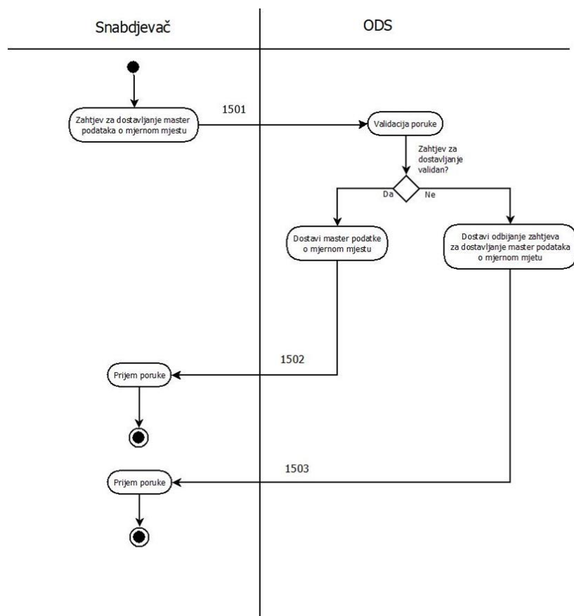
Slika 37: Dijagram aktivnosti za varijantu procesa Dostavljanje osnovnih (master) podataka snabdjevaču na njegov zahtjev
