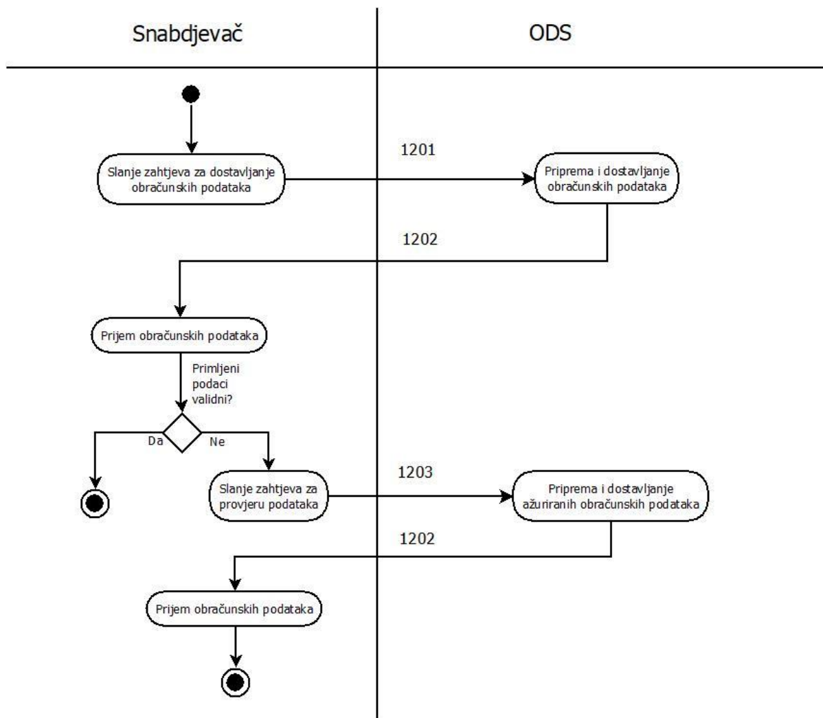
Slika 20: Dijagram aktivnosti procesa Dostavljanje obračunskih podataka snabdjevaču
