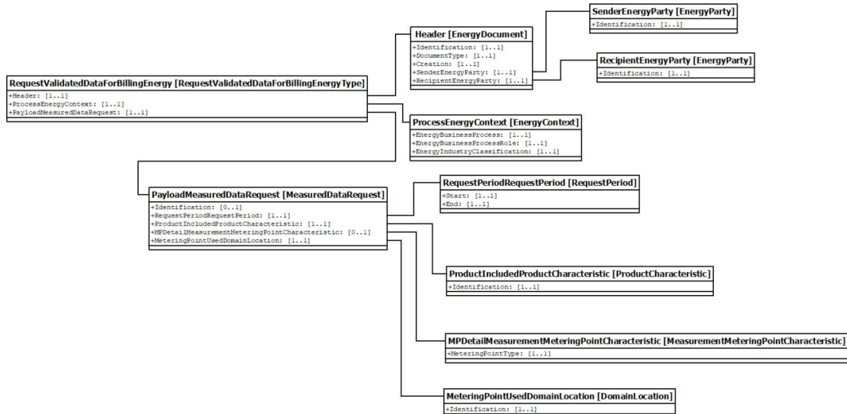
Slika 22: Dijagram klase za XML šemu RequestValidatedDataForBillingEnergy
