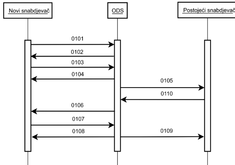
Slika 3: Sekvencijalni dijagram za proces Promjena snabdjevača RERS
