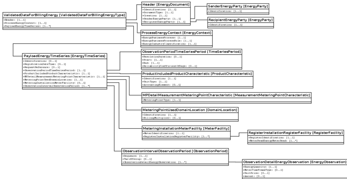
Slika 23: Dijagram klase za XML šemu ValidatedDataForBillingEnergy
