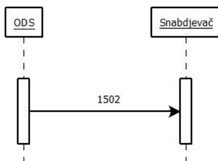
Slika 41: Sekvencijalni dijagram za varijantu procesa Dostavljanje osnovnih (master) podataka snabdjevaču samoinicijativno
