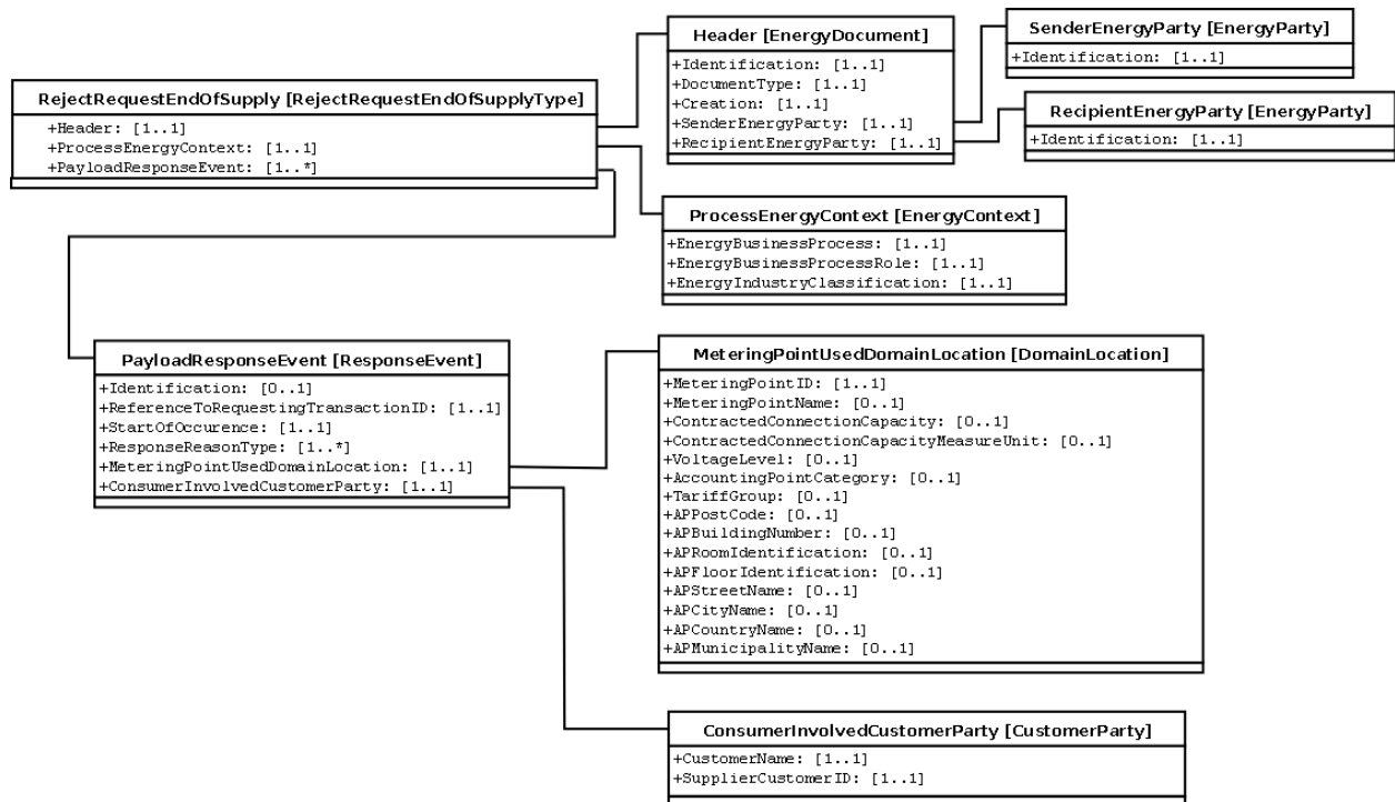
Slika 19: Dijagram klase za XML šemu RejectRequestEndOfSupply
