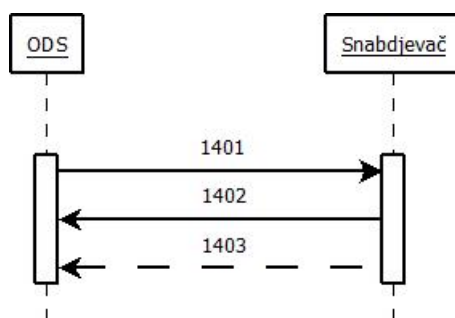
Slika 29: Sekvencijalni dijagram za proces Dostavljanja osnovnih (master) podataka ODS-u
