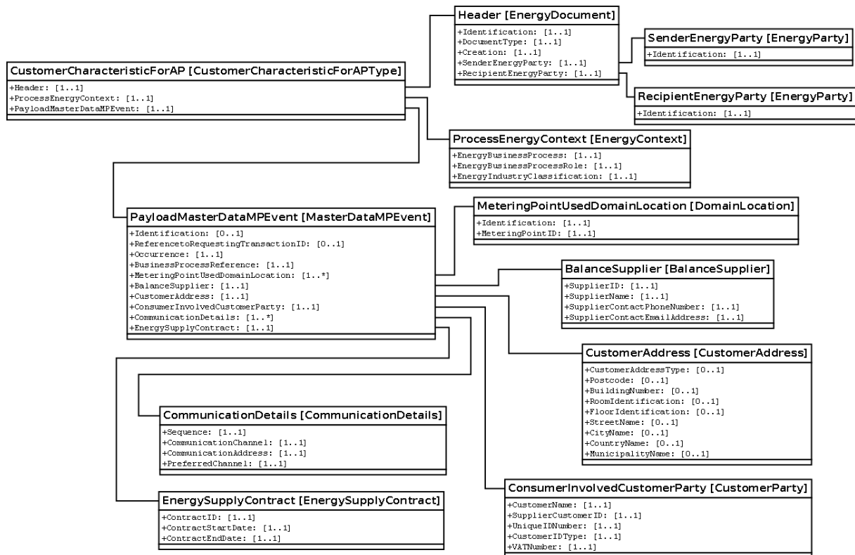
Slika 34: Dijagram klase za XML šemu CustomerCharacteristicsForAP
