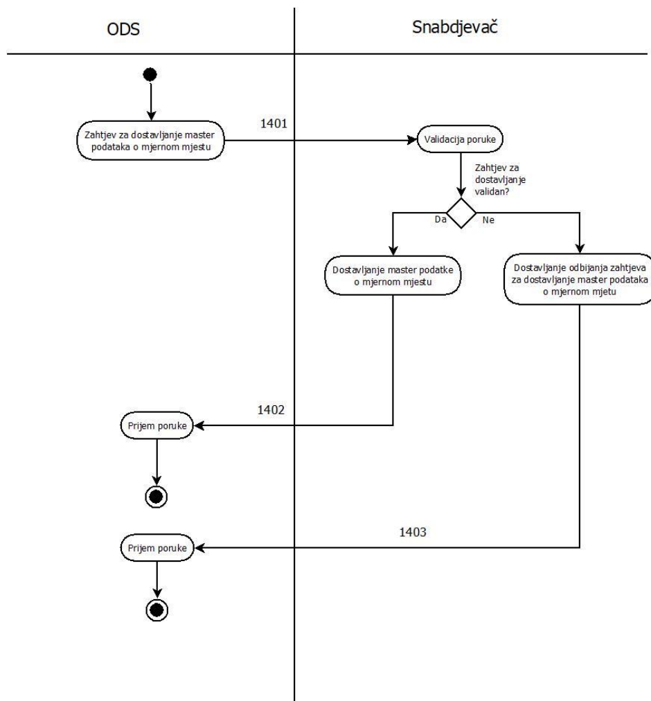
Slika 28: Dijagram aktivnosti procesa Dostavljanja osnovnih (master) podataka ODS-u
