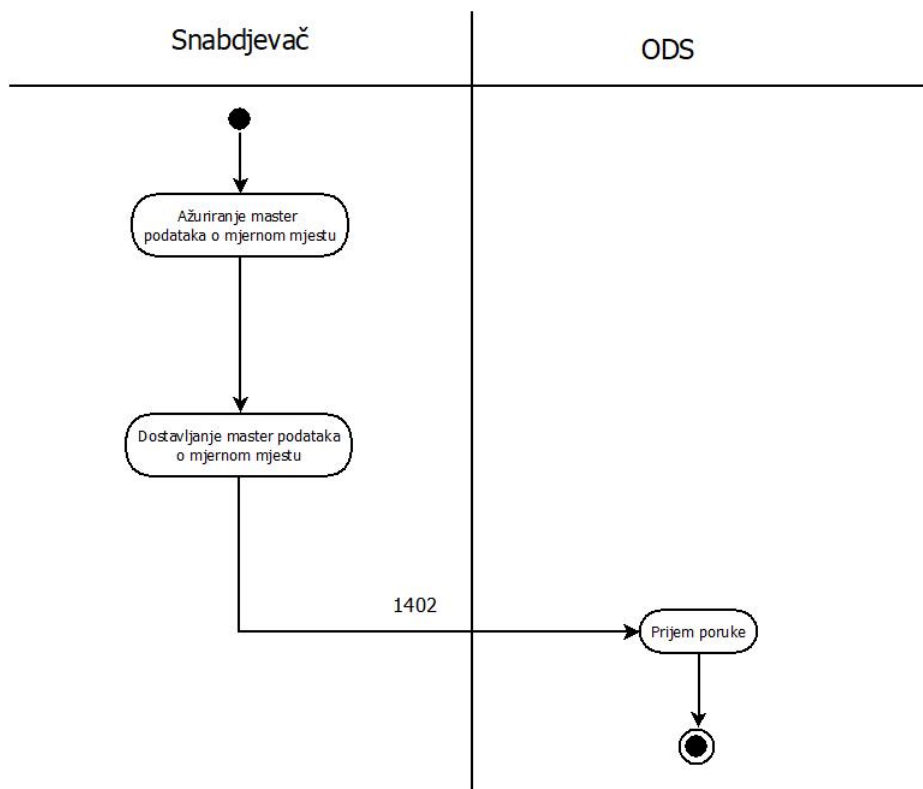
Slika 31: Dijagram aktivnosti varijante procesa Dostavljanja osnovnih (master) podataka ODS-u samoinicijativno
