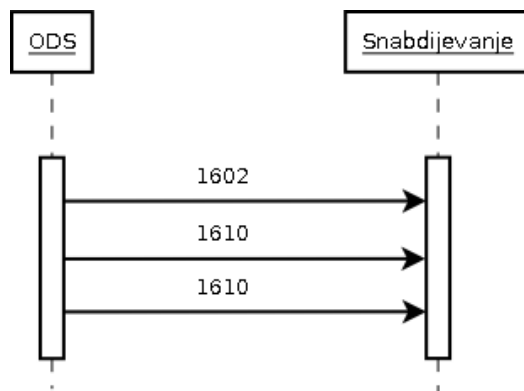
Slika 50: Sekvencijalni dijagram za varijantu procesa isključenja i uključanja mjernog mjesta koje pokreće ODS
