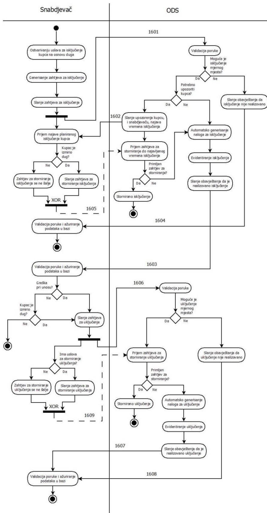
Slika 46: Dijagram aktivnosti za varijantu procesa Isključenja i uključjenja mjernih mjesta od strane ODS-a na zahtjev snabdjevača
