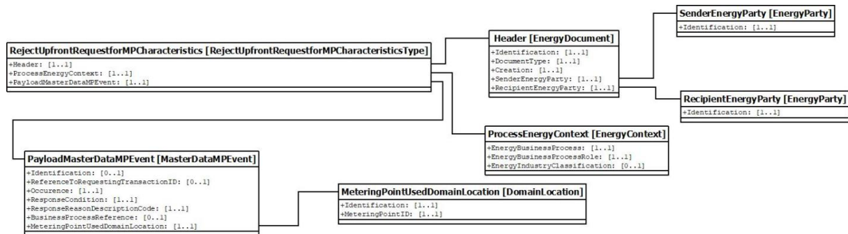
Slika 44: Dijagram klase za XML šemu RejectUpfrontRequestforMeteringPointCharacteristics
