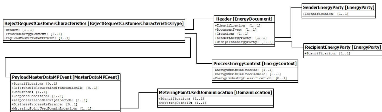
Slika 35: Dijagram klase za XML šemu RejectRequestCustomerCharacteristics
