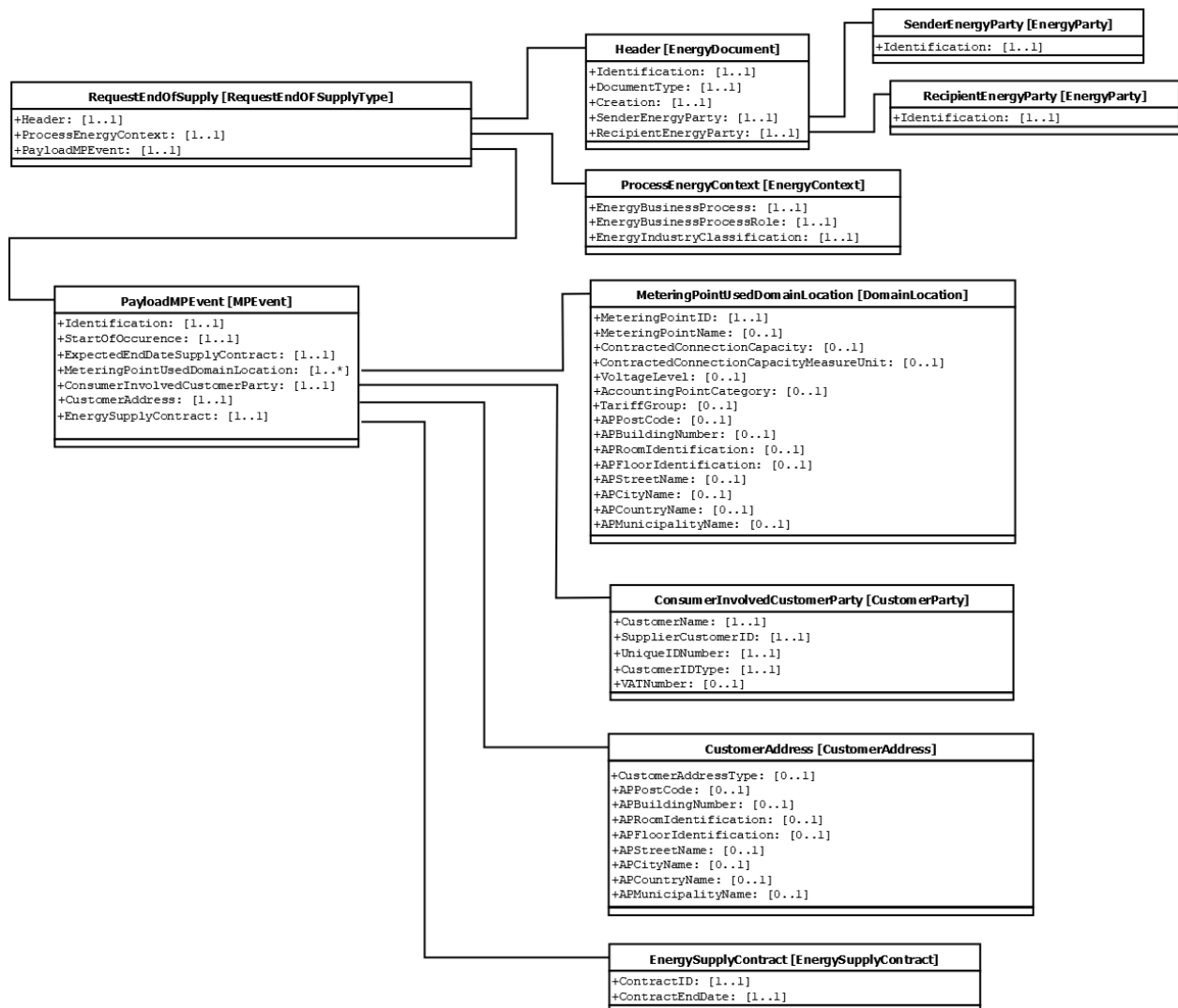
Slika 17: Dijagram klase za XML šemu RequestEndOfSupplier
