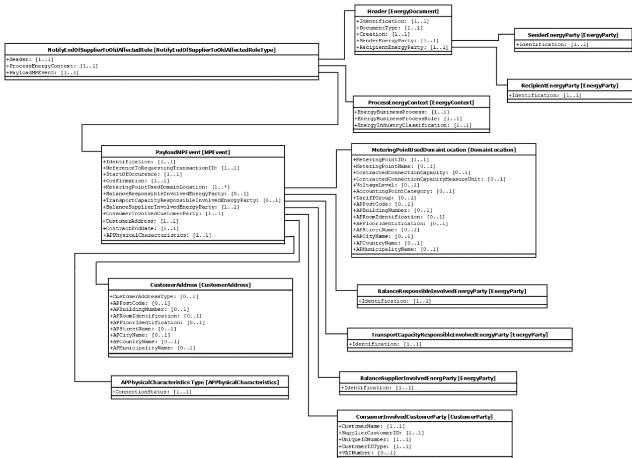
Slika 18: Dijagram klase za XML šemu NotifyEndOfSupplierToOldAffectedRole
