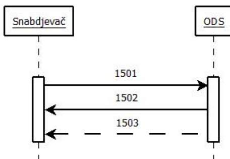
Slika 38: Sekvencijalni dijagram za varijantu procesa Dostavljanje osnovnih (master) podataka snabdjevaču na njegov zahtjev
