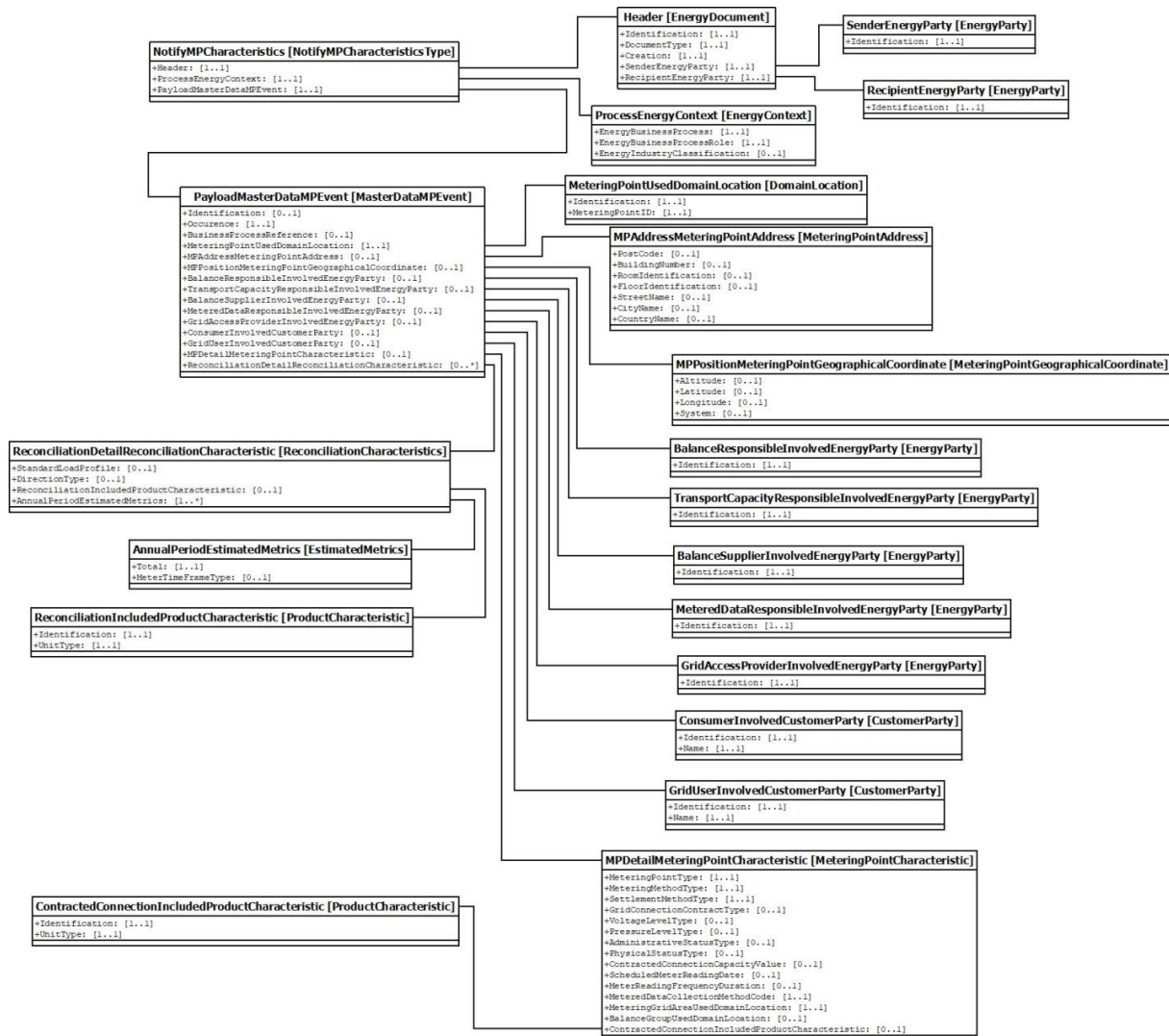
Slika 43: Dijagram klase za XML šemu NotifyMPCharacteristics
