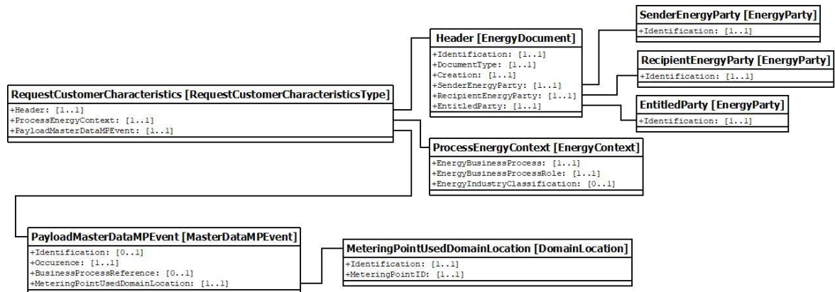
Slika 33: Dijagram klase za XML šemu RequestCustomerCharacteristics
