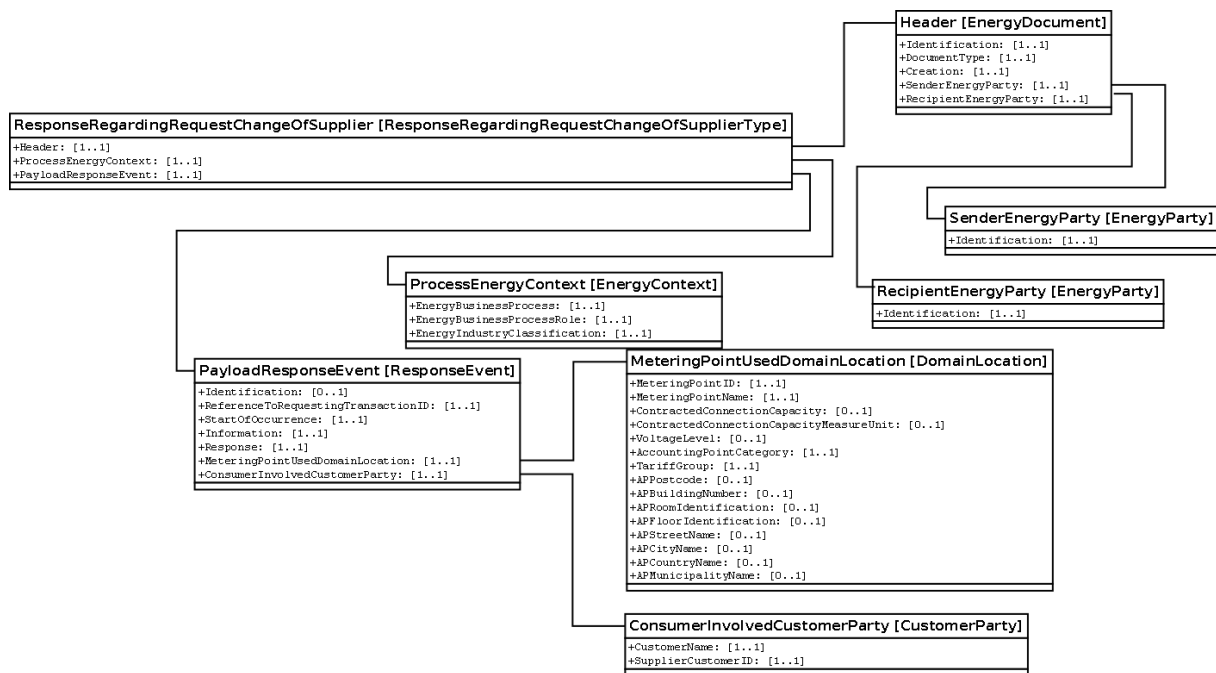
Slika 13: Dijagram klase za XML šemu ResponseRegardingRequestChangeOfSupplier
