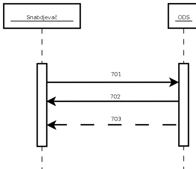
Slika 16: Sekvencijalni dijagram za proces Raskida ugovora o snabdijevanju RERS
